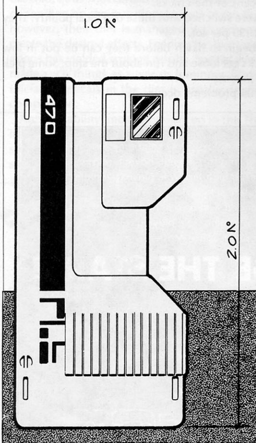
STOWED CONFIG. 2.0M x 1.0M x 0.5M
