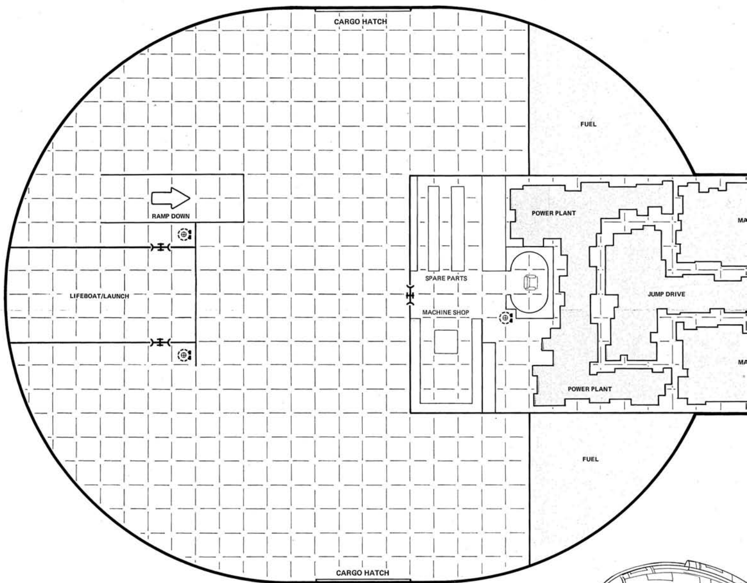
TWEEN DECK
